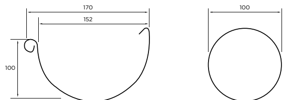
Sistem pluvial mare 165/100 mm
